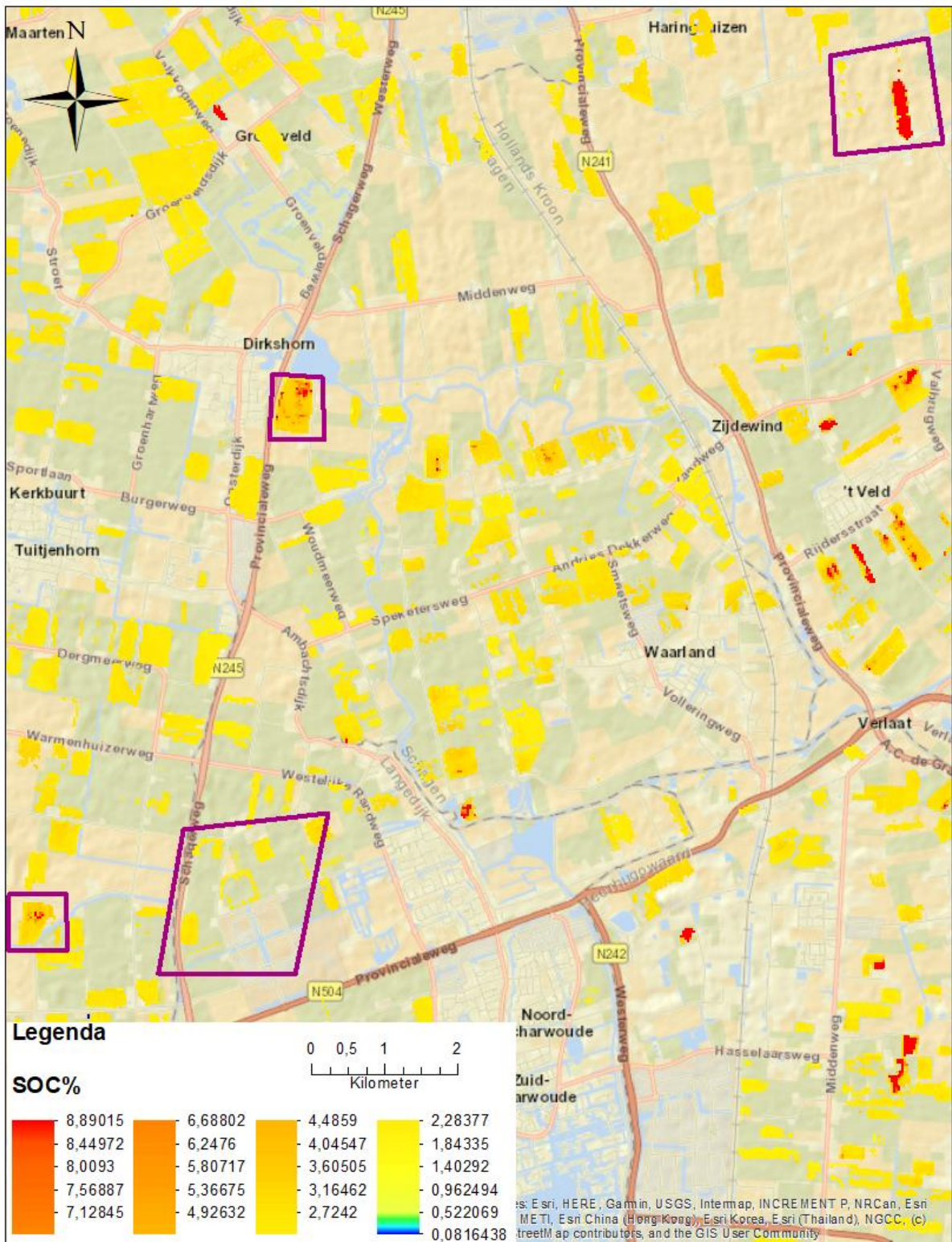
Figuur 21: Voorspelling SOC% door Sentinel-2, Noord-Holland. De polygoenen getekend in de afbeelding zijn de geselecteerde percelen voor validatie van de voorspelling van organische koolstofpercentage door Sentinel-2. In deze afbeelding zijn niet alle geselecteerde percelen voor validatie opgenomen.
