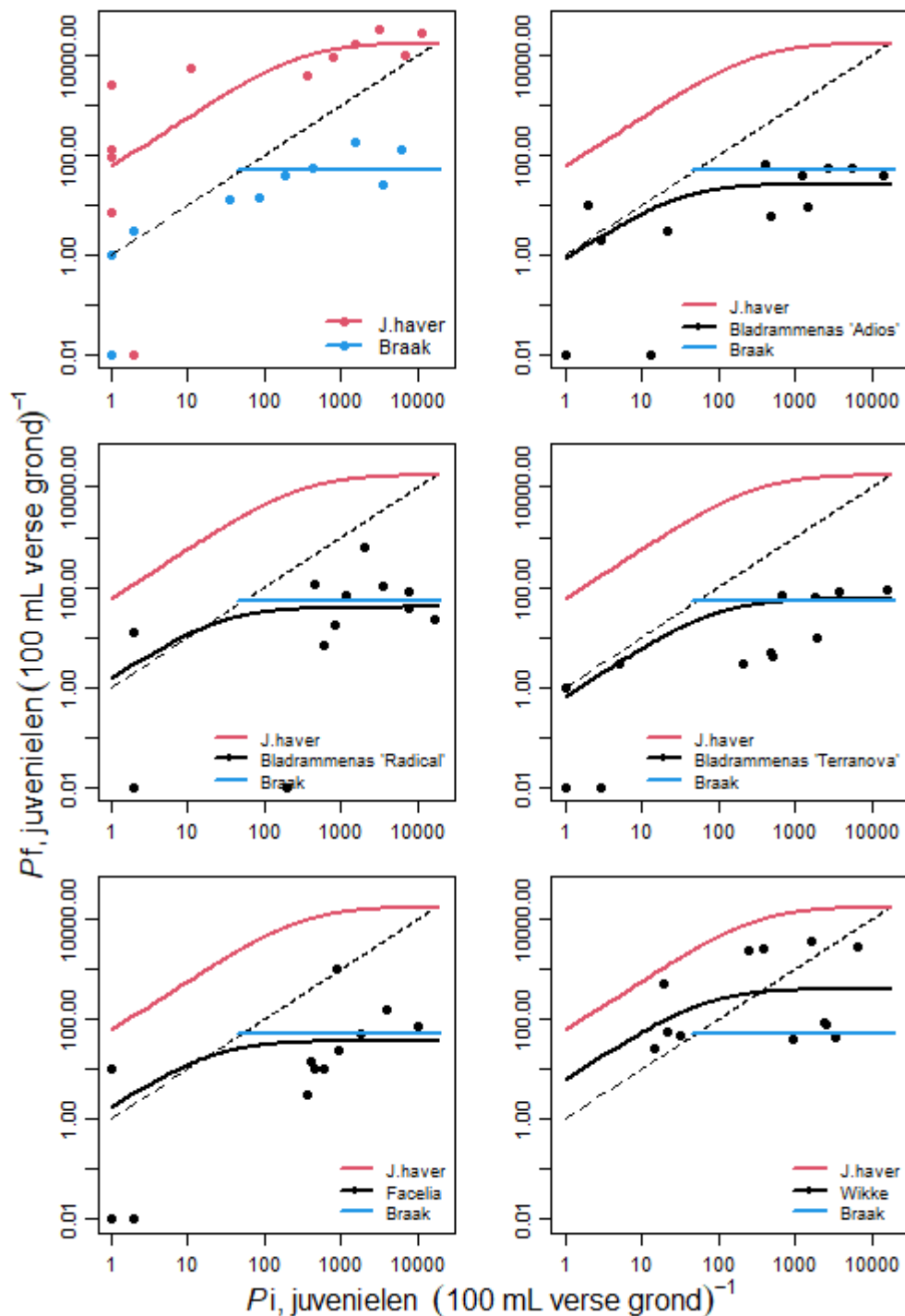
Figuur 9a. Gemeten P_i - en P_f -waarden van M. chitwoodi en gefitte Seinhorstcurves voor zes groenbemesters en vier mengsels (van twee groenbemesters) die geoogst zijn in december 2019. De P_i is bepaald in augustus 2019. De lijn voor braak is de gemiddelde P_f -waarde bij P_i -waarden > 50. Wanneer de gemeten P_f -waarde gelijk was aan 0 is deze vervangen door 0.01 om te kunnen weergegeven op logaritmische schaal. Stippellijn: einddichtheid is gelijk aan de begindichtheid.
