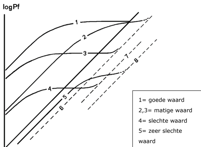
Figuur 2. Schematische weergave van de relatie tussen begin ( P_i )- en eindbesmetting ( P_f ) bij verschillende waardgewassen. (Seinhorst, 1970, Schomaker, 2013)
