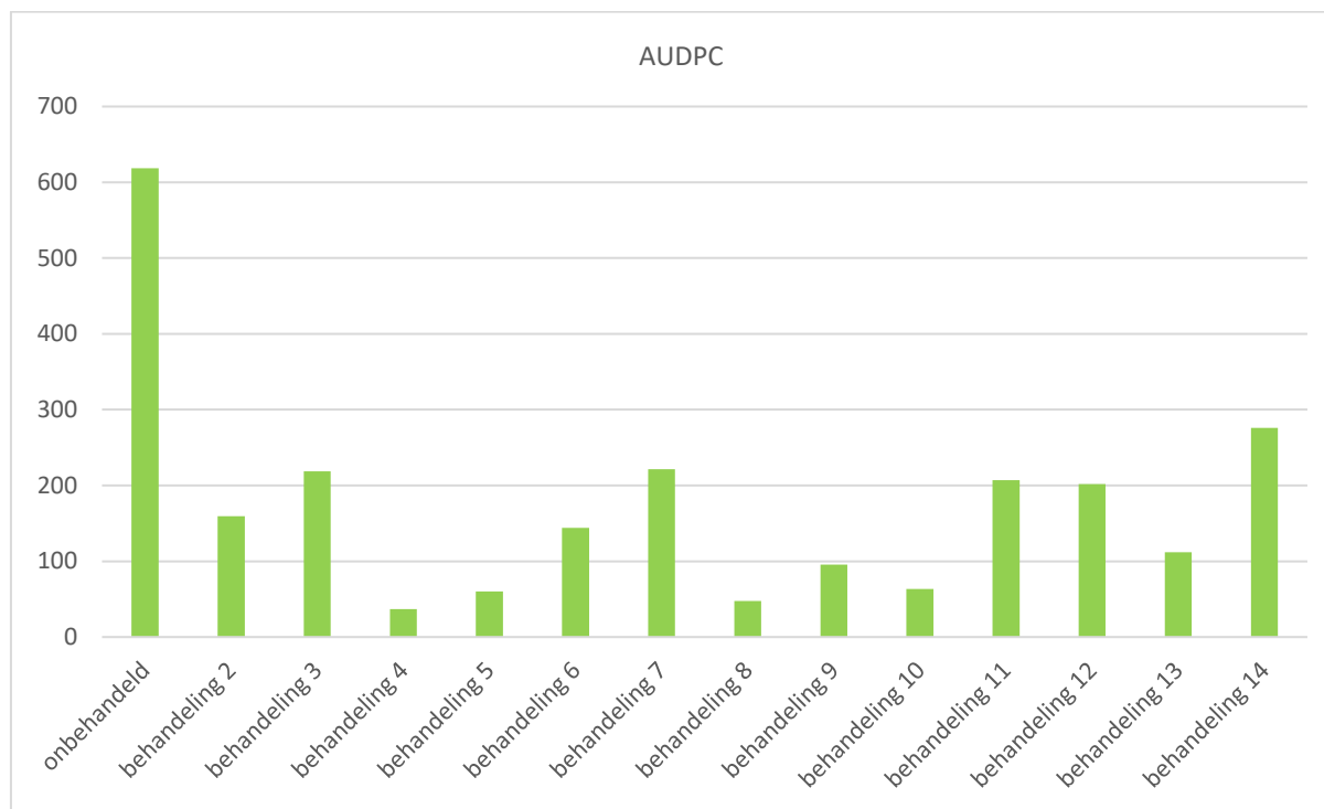
Grafiek 3. AUDPC
