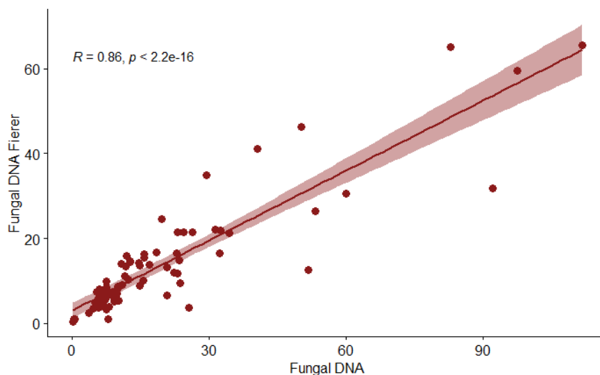
Fig. 3.10: Correlatie tussen DNA concentratie (pg/μl) gemeten met de Fierer primers en de 5.8S-Fun en de ITS4-Fun primers.
